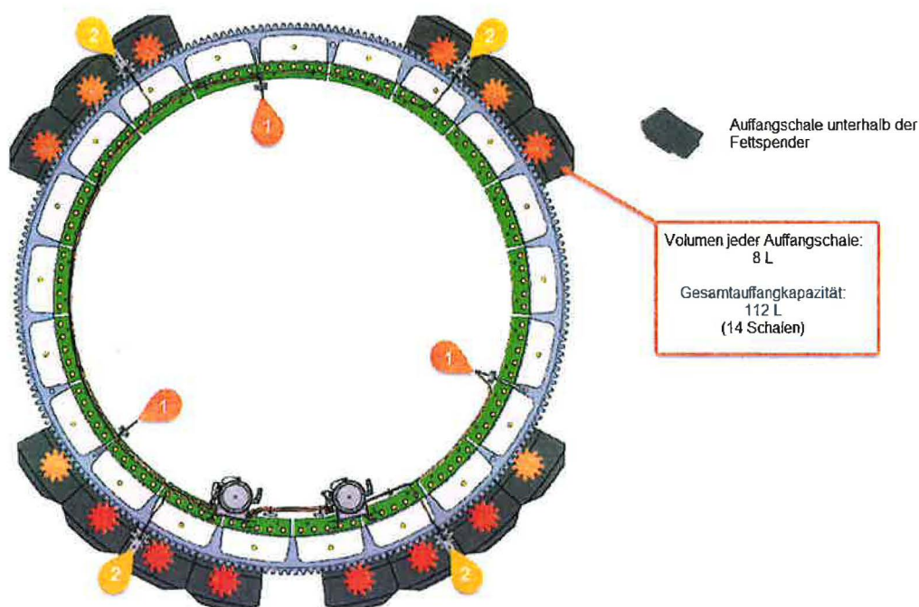
Abbildung 3: Auffangschalen am Azimutgetriebe
