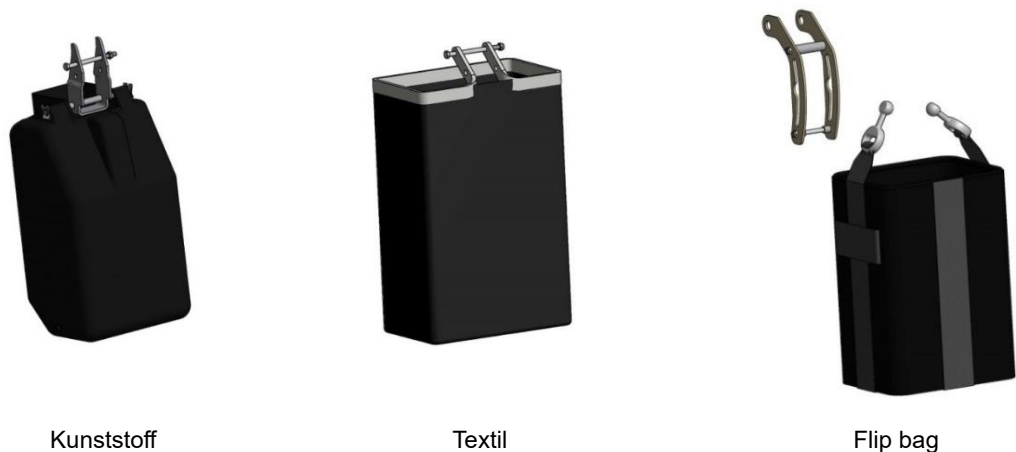
Bild 10: Kettenspeichertypen
