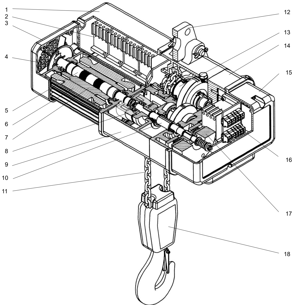
Bild 2: Schnittbild
