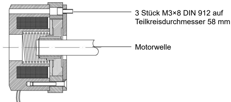
Bild 29: Aufbau der Fahrwerksbremse Typ BFK
