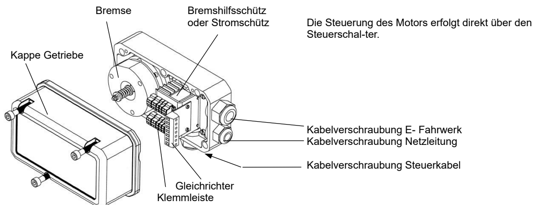
Bild 17: Direktsteuerung
