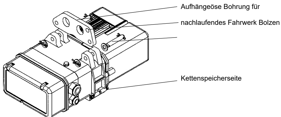
Bild 6: Aufhängung mit Aufhängeöse
