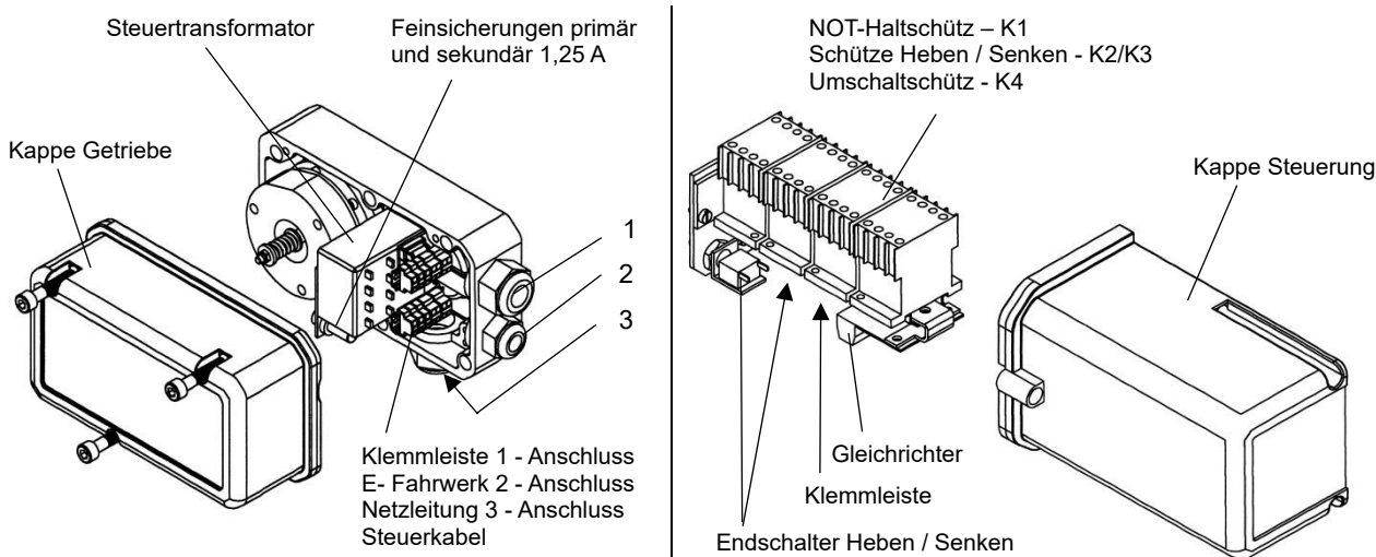
Bild 18: Schützsteuerung
