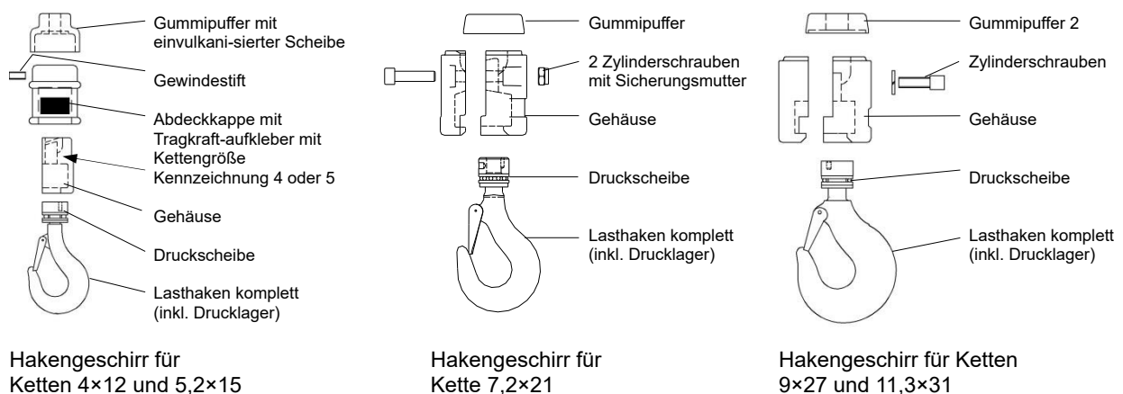
Bild 4: Aufbau der Hakengeschildre
