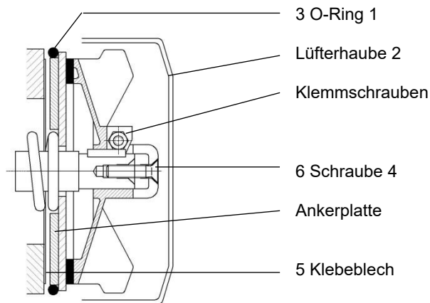
Bild 30: Aufbau der Fahrwerksbremse Typ EFB
